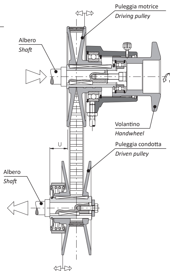
MONTAGGIO A "U" - "U" ASSEMBLY
