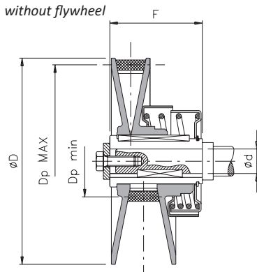
VAR.D.E.A.C./TE/IF/S versione senza volantino without flywheel
