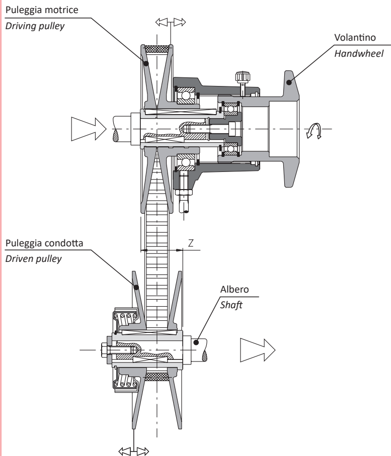
MONTAGGIO A "Z" - "Z" ASSEMBLY
